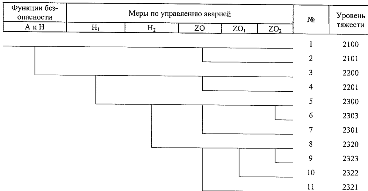
Рисунок 5. Обобщенное дерево событий для аварий с большим и средним нарушением целостности границы первого контура в пределах ГО
